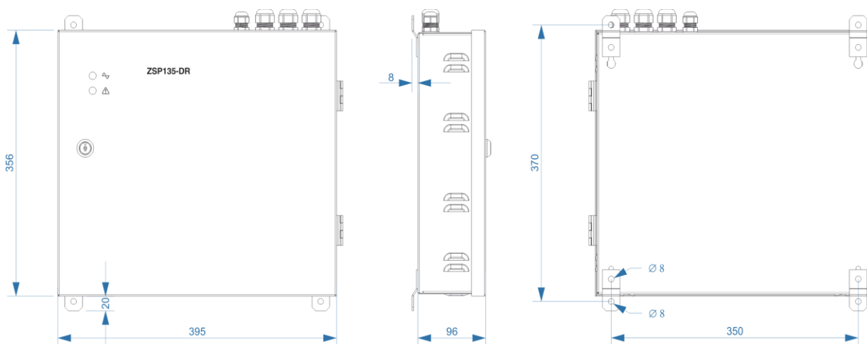
Rys. 1. Widok, wymiary gabarytowe i rozmieszczenie otworów mocujących dla przykładowego zasilacza ZSP135-DR-5A-1.
