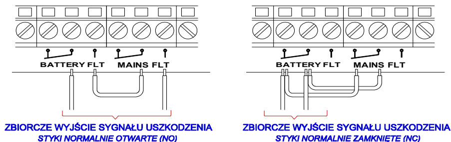
Rys. 3. Konfiguracja zbiorczego sygnału o uszkodzeniu
