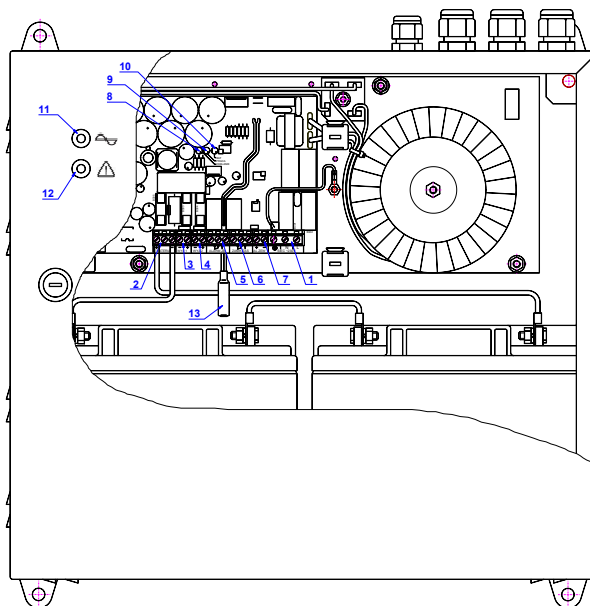
Rys. 2. Widok zasilacza ZSP135-DR.
