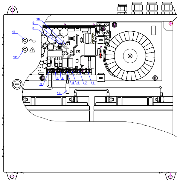
Abb. 2 Ansicht des Netzteils ZSP135-DR.
