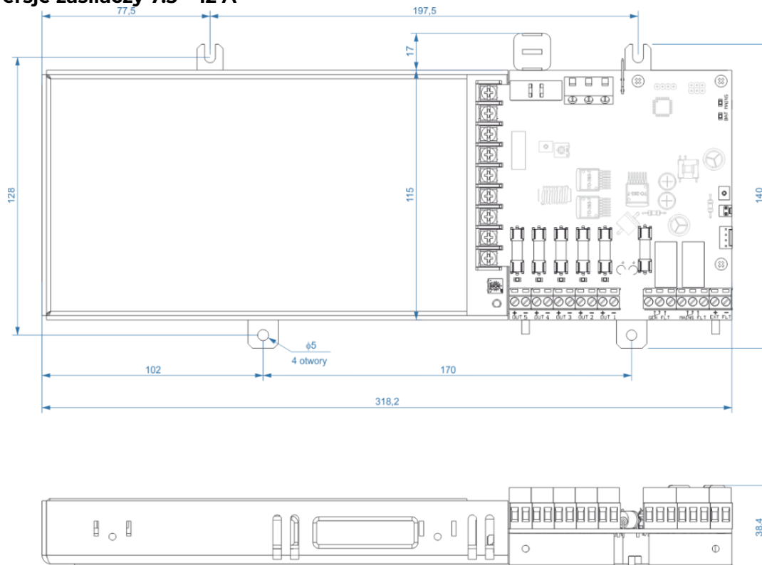
Rozmieszczenie otworów mocujących i wymiary zewnętrzne zasilaczy ZSPM-200 i ZSPM-320.
